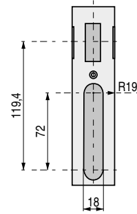
Detalle regulación del picaporte y cajetín de protección
