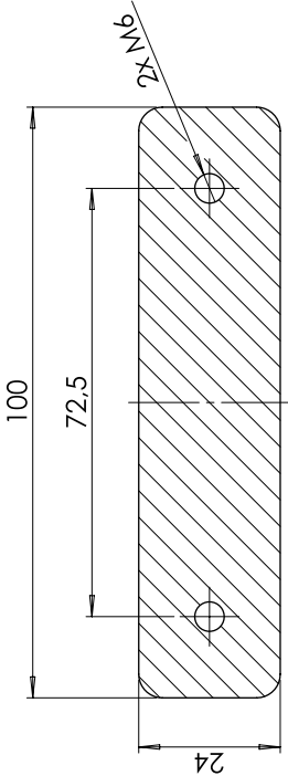
SCHNITT A-A 1 : 1
