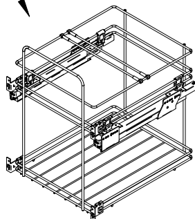
PKBGM453M 30L+10L+9L
