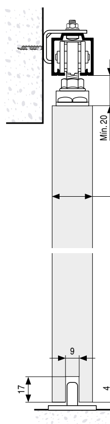
Aplicación NK 50 Superior con perfil y escuadra a la pared
