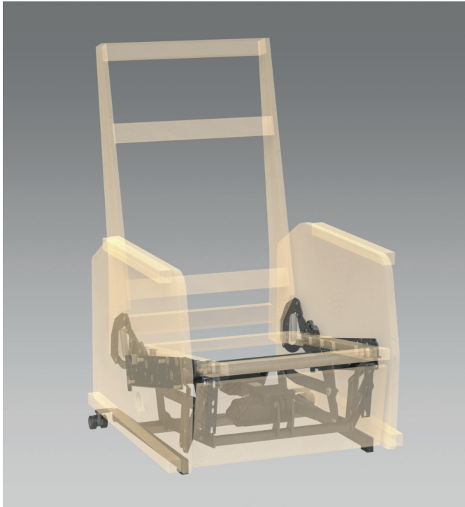
Mecanismo con 1 motor
