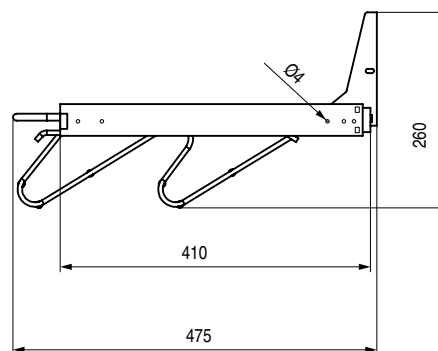
VISTA PERFIL
